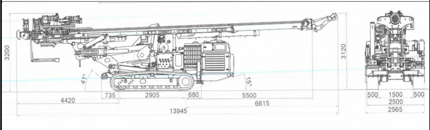
Rig Dimensions
